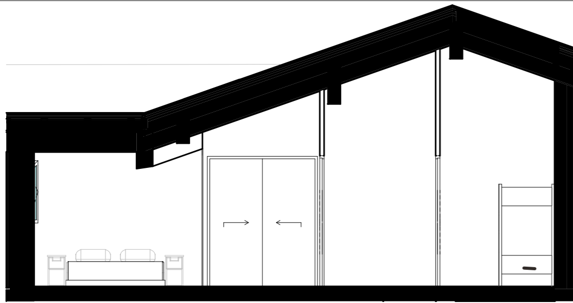
Coupe Y1008
