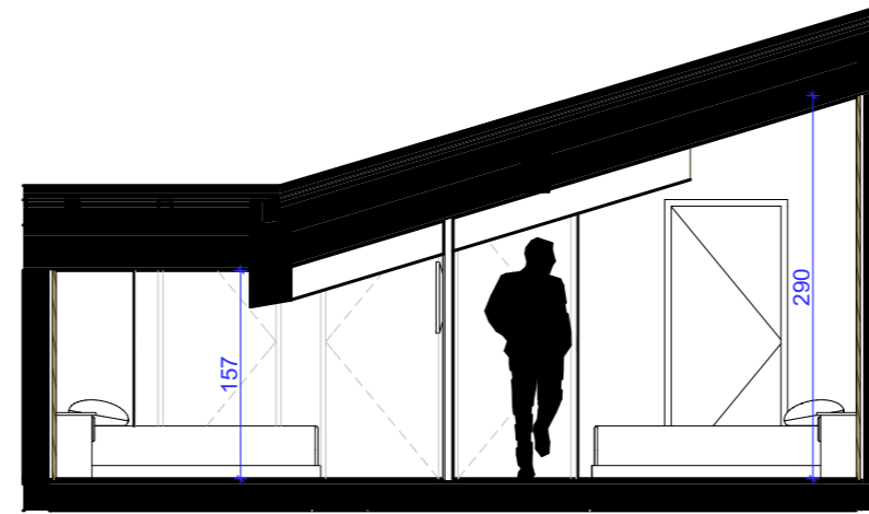
Coupe X1007
