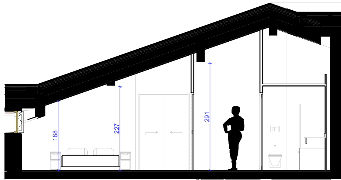
Coupe Y1007
