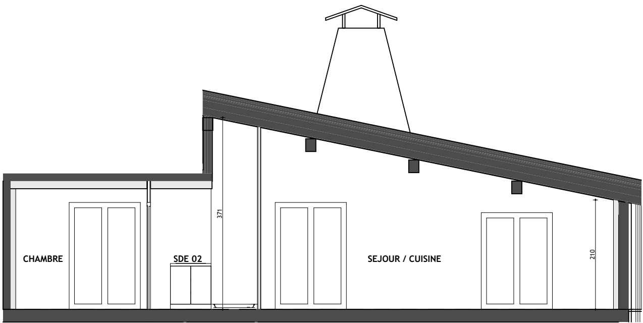
coupe
