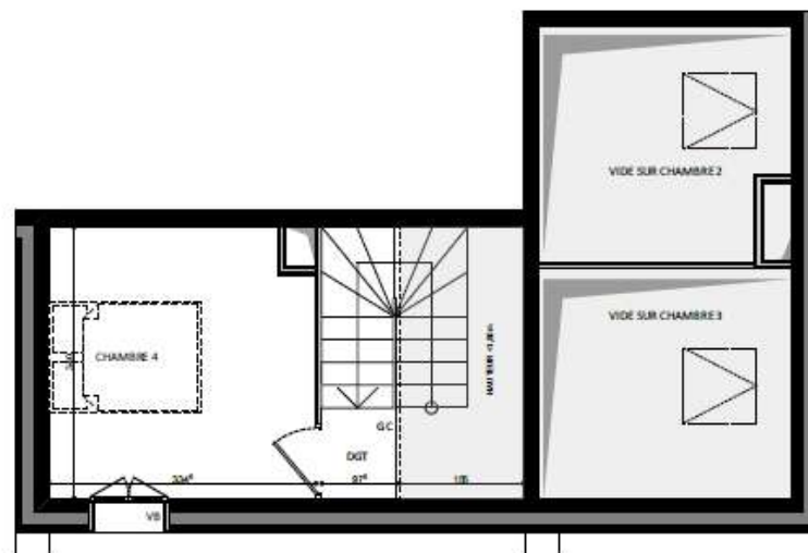
NIVEAU COMBLES 2
