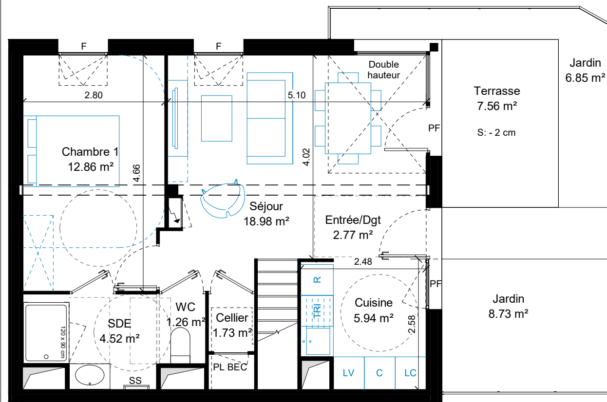
PLAN RDC
